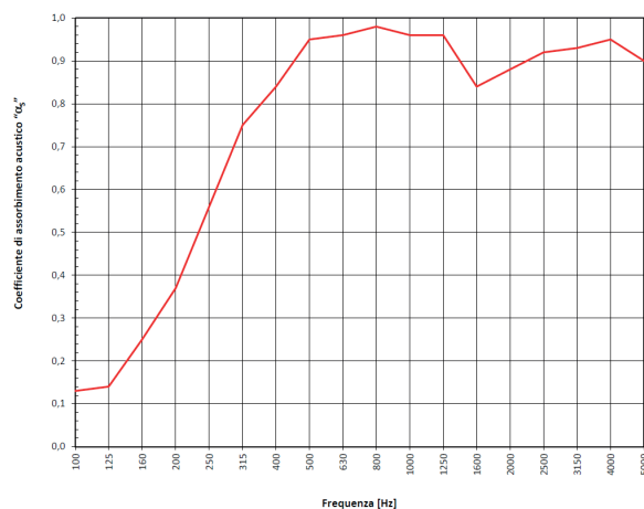
ANDAMENTO DEL COEFFICIENTE DI ASSORBIMENTO ACUSTICO "α w " PER TERZI D'OTTAVA
