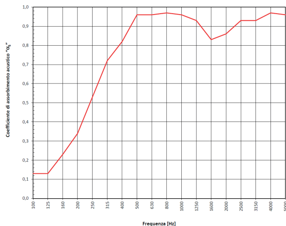
ANDAMENTO DEL COEFFICIENTE DI ASSORBIMENTO ACUSTICO "α s " PER TERZI D'OCTAVA
